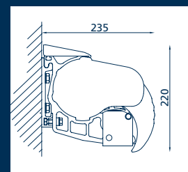
Montaggio a parete con terminale 31592 Wall installation with 31592 terminal bar
