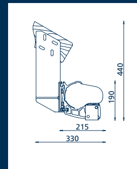
Montaggio sottotetto Under-roof installation
