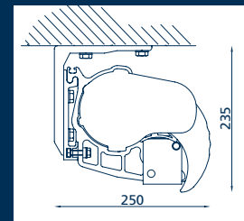
Montaggio a soffitto con terminale 31592 Ceiling installation with 31592 terminal bar
