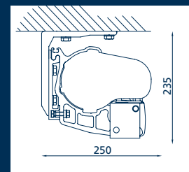
Montaggio a soffitto Ceiling installation
