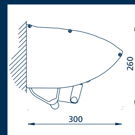
Montaggio con tettuccio Installation with a hood
