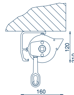
Ingombri cassonetto Boxe encumbrance
