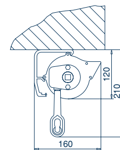
Ingombri cassonetto Boxe encumbrance
