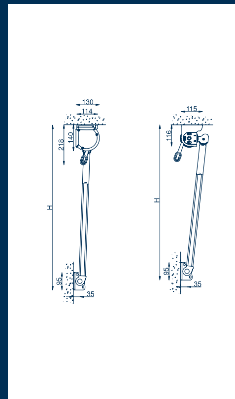
Montaggio a soffitto Ceiling installation
